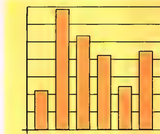
Ступінчастий графік, застосовується для порівняння залежностей різних величин
